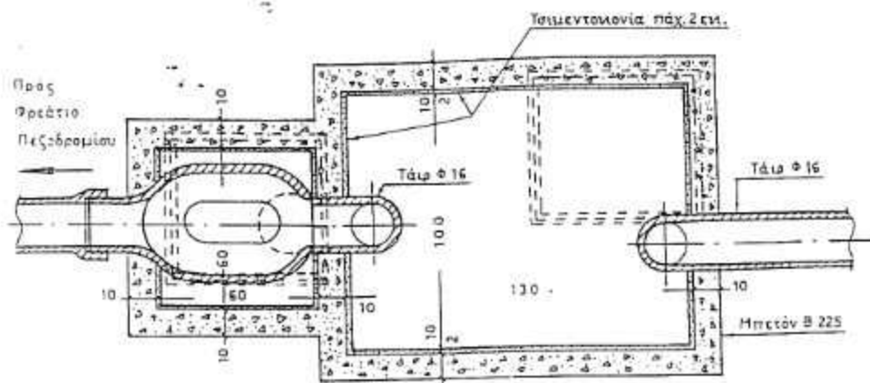
ΚΑΤΟΨΗ. ΚΛ.1:20.
