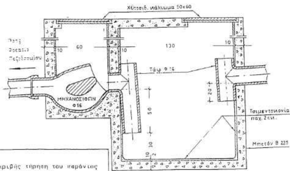
ΤΟΜΗ. ΚΛ.1:20.
